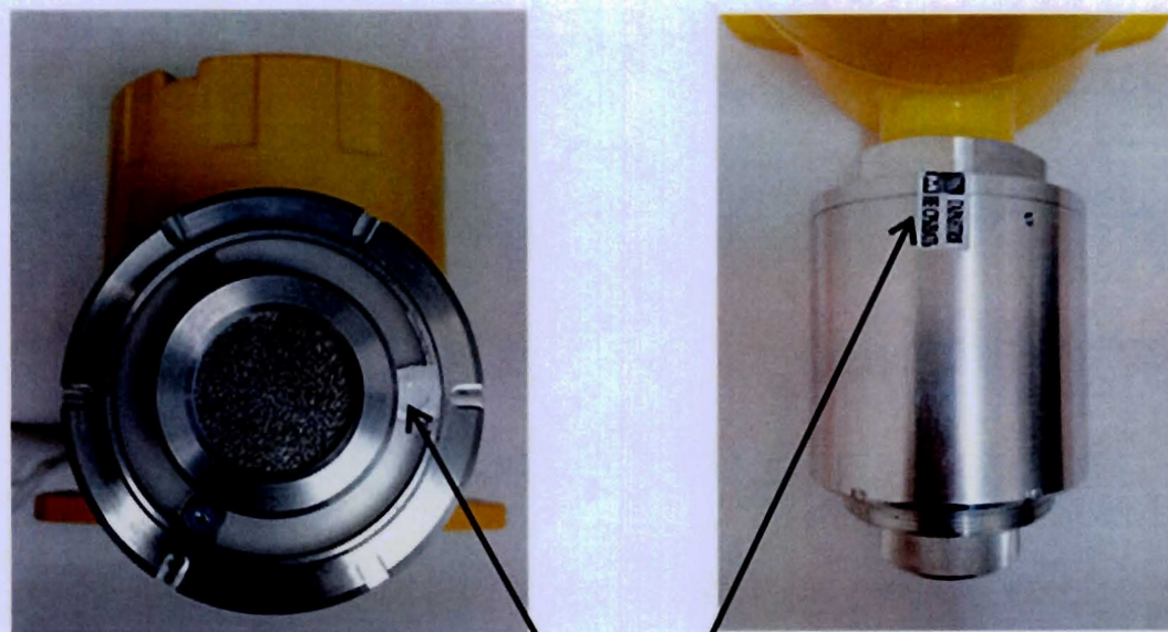
Место нанесения пломбы для ИГМ-12
