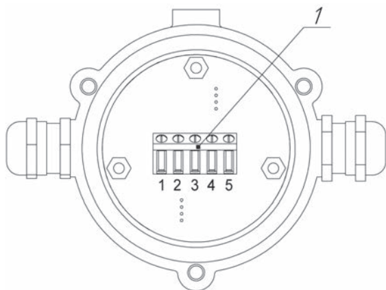
1- Клеммная колодка
